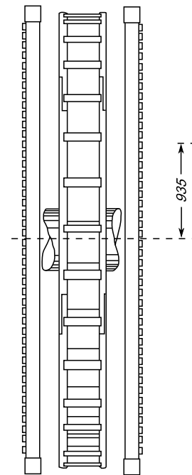
Rekonstruktion des Wasserrades der Hütte am Alzendeich Basierend auf den Zeichnungen von Albert Knaff aus dem Jahre 1910 Neu gezeichnet und tlw. berichtigt März 2008 durch Marcel Normann
