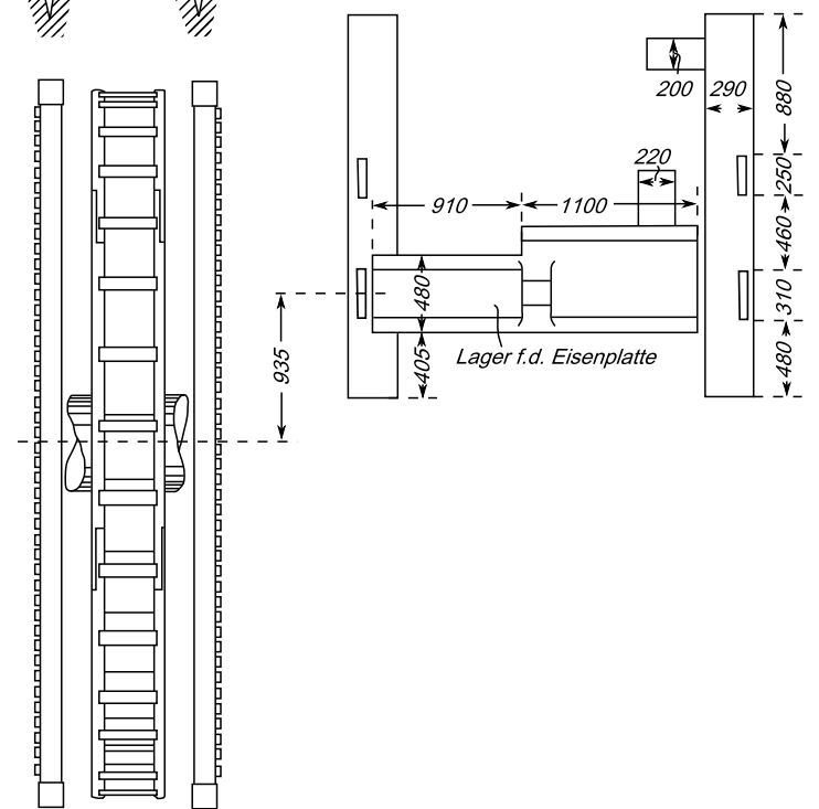
Rekonstruktion des Wasserrades der Hütte am Alzendeich Basierend auf den Zeichnungen von Albert Knaff aus dem Jahre 1910 Neu gezeichnet und tlw. berichtigt März 2008 durch Marcel Normann
